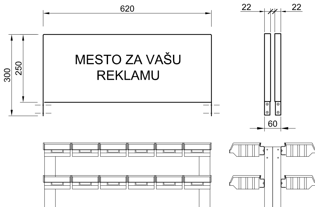
reklamni pano i stojeći nosač pre montaže
